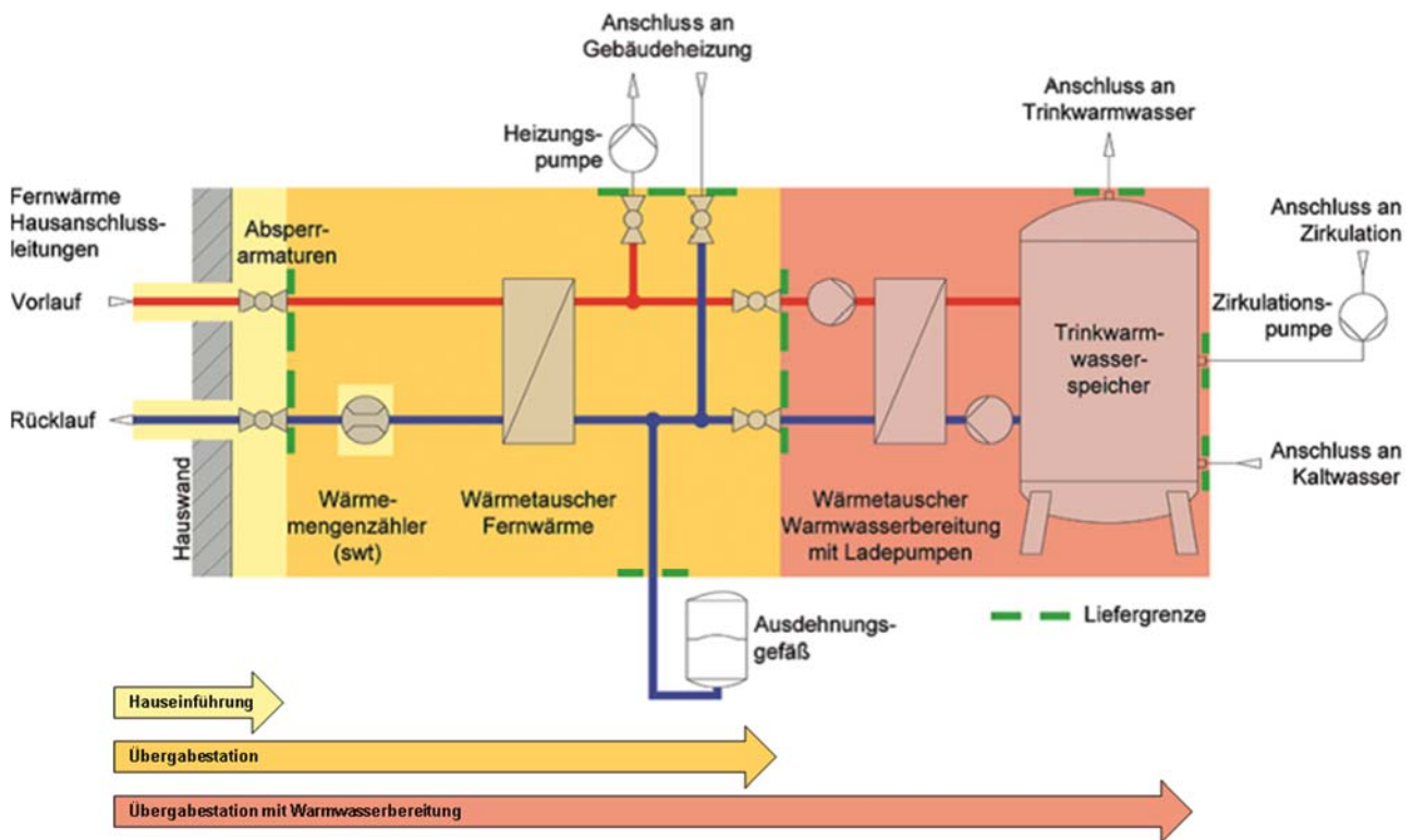
Abbildung 9: Leistungs-, Liefer- und Eigentumsgrenzen
