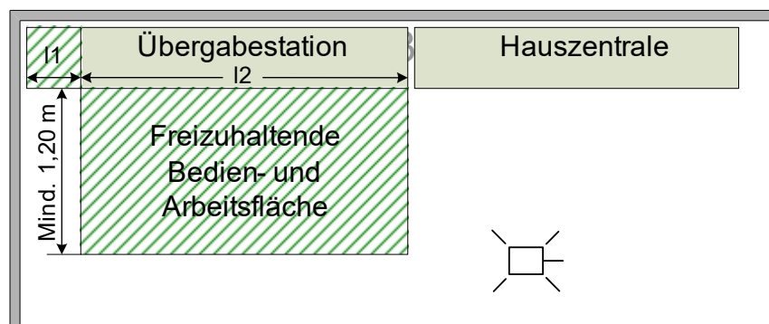
Abbildung 6: Hausanschlusswand
