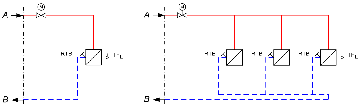
Abbildung 11: Hauszentrale-Raumluftheizung Prinzipschaltbilder für den indirekten Anschluss
