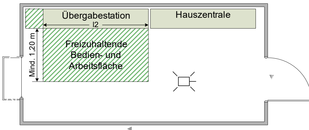
Abbildung 5: Hausanschlussraum
